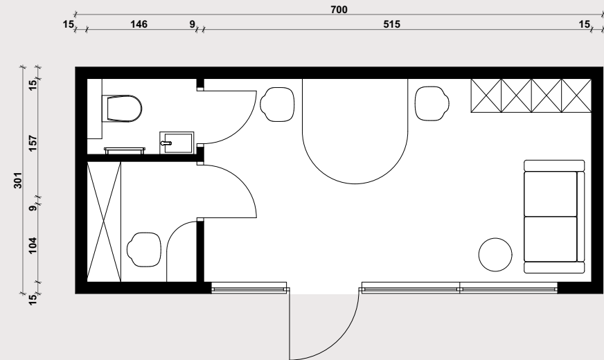
Sanitäranlage Beispielgrundriss
