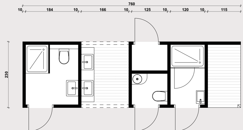
Sanitäranlage Beispielgrundriss
