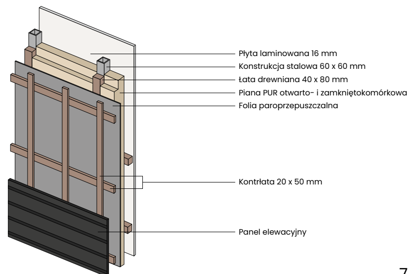
Przekrój ściany
