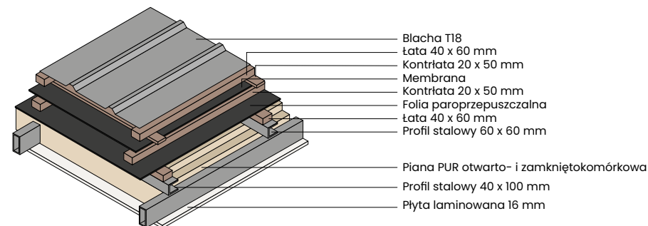
Przekrój podłogi
